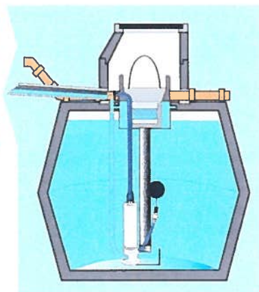
Installationsschema mit Unterwasserpumpe COMBIPRESS
