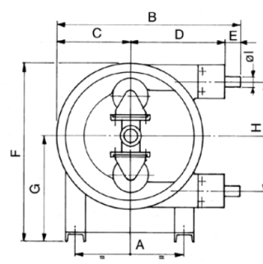
ASP 25 - 32 - 40 - 50 - 65 FX
