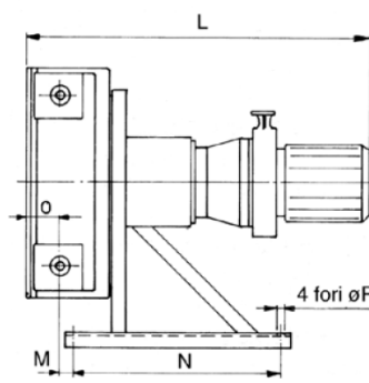
ASP 25 - 32 - 40 - 50 - 65 FX
